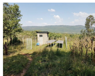
L'impianto di irrigazione alimentato da energia solare realizzato in Wolaita, Sud Etiopia
